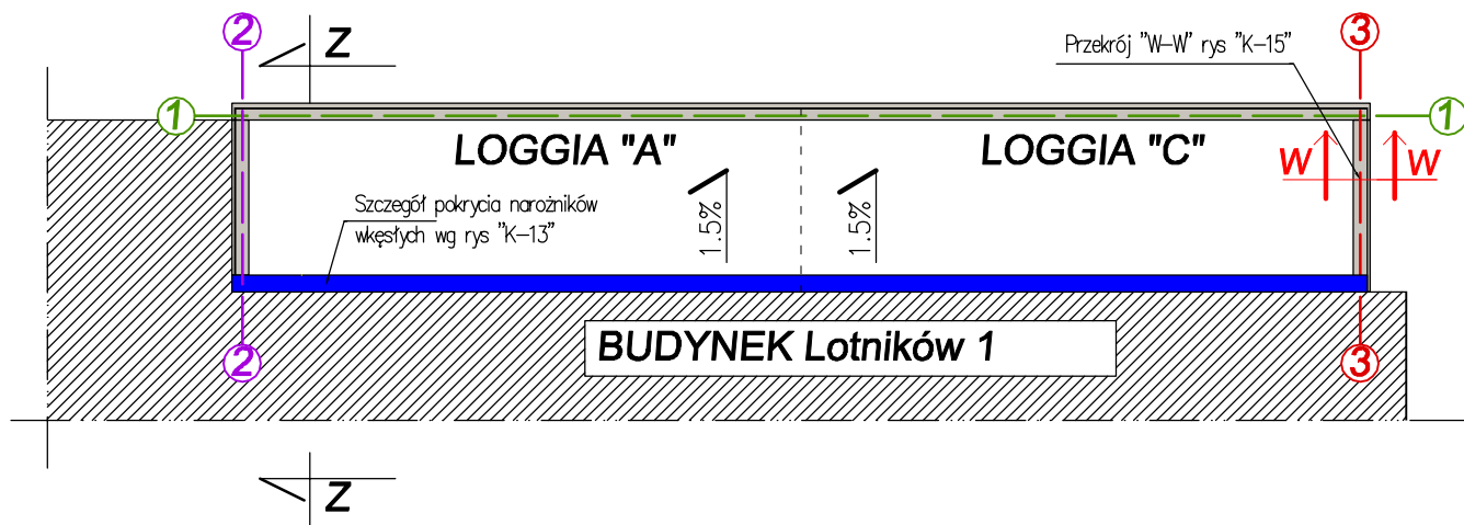
OPIERZENIE linia "1-1" blacha aluminiowa gr.1mm
