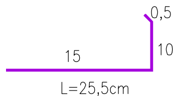
OPIERZENIE linia "3-3" blacha aluminiowa gr 1,0 mm
