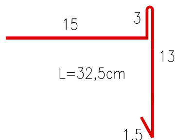
OPIERZENIE linia "3-3" blacha aluminiowa gr 1,0 mm
