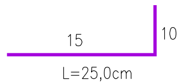
OPIERZENIE linia "2-2" blacha aluminiowa gr 1,0 mm
