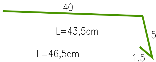
OPIERZENIE linia "1-1" blacha aluminiowa gr.1,0 mm
