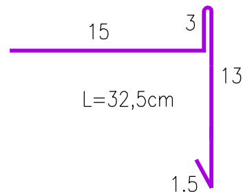
OPIERZENIE linia "2-2" blacha aluminiowa gr 0.5mm
